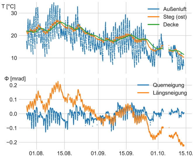
Bild 10: Messdatenverlauf über zweieinhalb Monate; oben: ausgewählte Temperaturen und unten ambiante Neigungen (1 Datenpunkt pro 10 Minuten)
