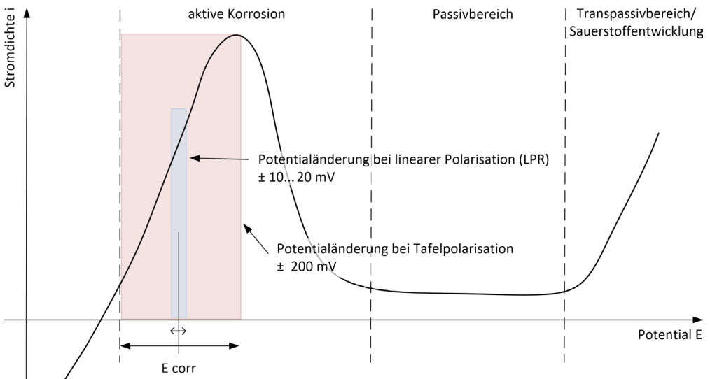
Bild 5: Stromdichte-Spannungskurve von Stahl mit Darstellung des Aktiv- und Passivbereichs sowie der Arbeitsbereiche für lineare Polarisation und Tafelpolarisation
