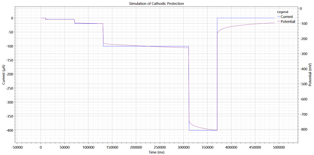
Bild 10: Beispiel für eine galvanostatische Simulationsmessung für KKS (hier mit anderen Pulszeiten für die Polarisationsstufen)
