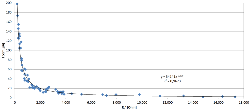
Bild 9: Grafischer Zusammenhang zwischen Datenpaaren I_{corr} aus Tafel-Polarisation und R_p aus LPR aus Messungen von sechs verschiedenen Praxisprojekten, aus [4]
