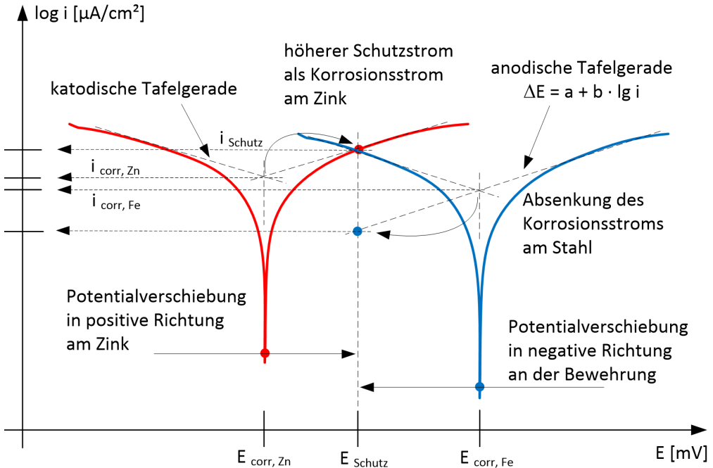
Bild 2: Wirkungsprinzip des galvanischen KKS mit Zink für Stahl in der Stromdichte-Spannungs-Darstellung, nach [3]
