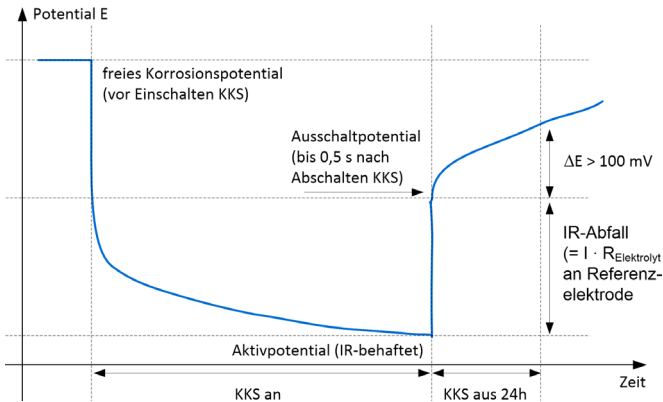
Bild 1: Darstellung des Potentialverlaufs sowie des IR-Abfalls als Messeffekt an der Referenzelektrode unter KKS und während der Depolarisationsmessung
