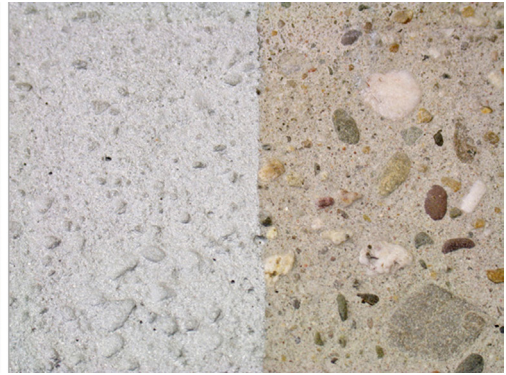
Bild 3: Thermisches Spritzverzinken von Beton – händisches Spritzen und Ansicht der verzinkten/unverzinkten Betonoberfläche (Abbildungen: Grillo Werke AG)
