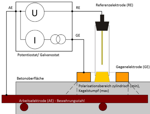
Bild 6: Prinzipskizze für Potentiostat und Messanordnung sowie Beispiel für praktische Anwendung in einem Parkhaus (Aufsatzmesszelle links unten)
