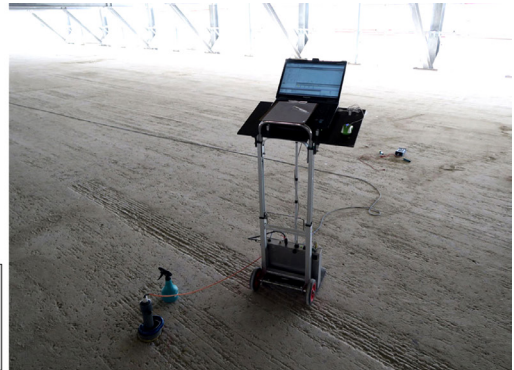
Bild 6: Prinzipskizze für Potentiostat und Messanordnung sowie Beispiel für praktische Anwendung in einem Parkhaus (Aufsatzmesszelle links unten)
