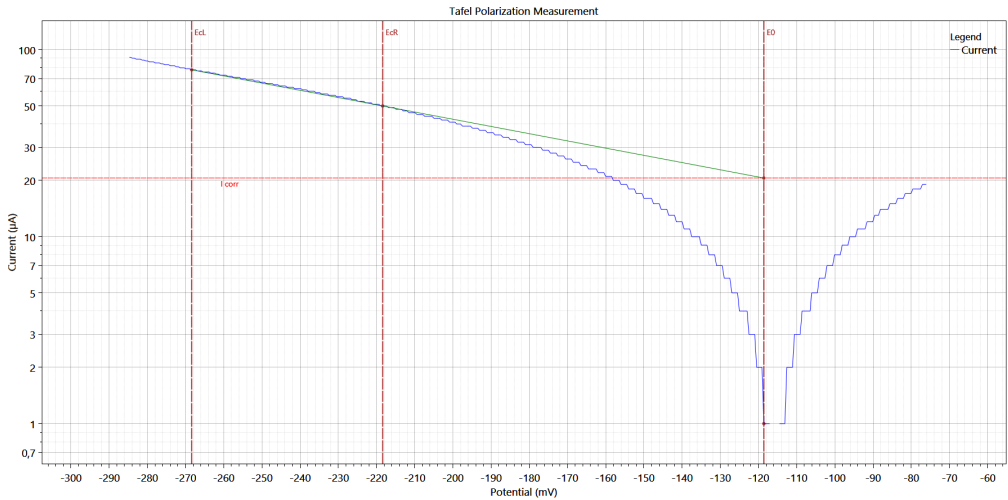
Bild 8: Beispiel für Tafel-Polarisationsmessung mit vertikalen Linien E_{cl} und E_{cr} zum Anfinden der Tafel-Geraden und deren Schnittpunkt mit E_0 , an dem der Korrosionsstrom am Korrosionspotential abgelesen werden kann
