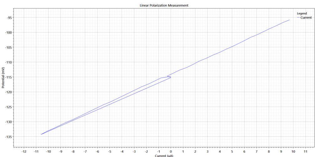
Bild 7: Beispiel für lineare Polarisationsmessung mit exakt linearem Bezug zwischen Potential und Strom innerhalb der Versuchsgrenzen
